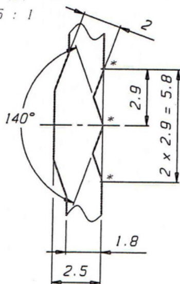
Szczegół "B"
